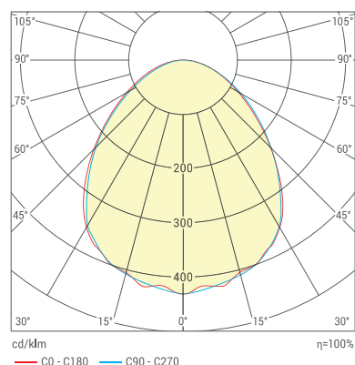
КСС (микропризма)
